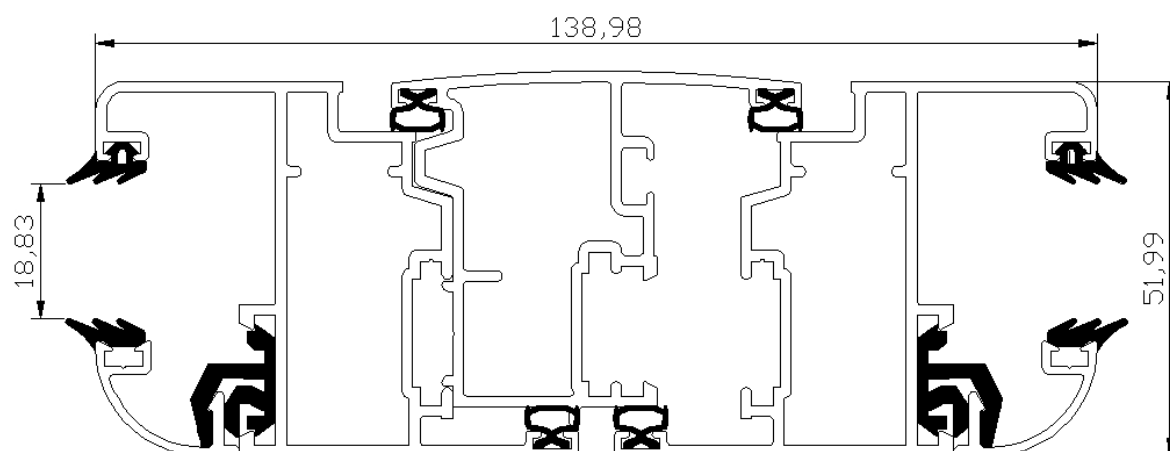
Sección A22 CENTRAL
